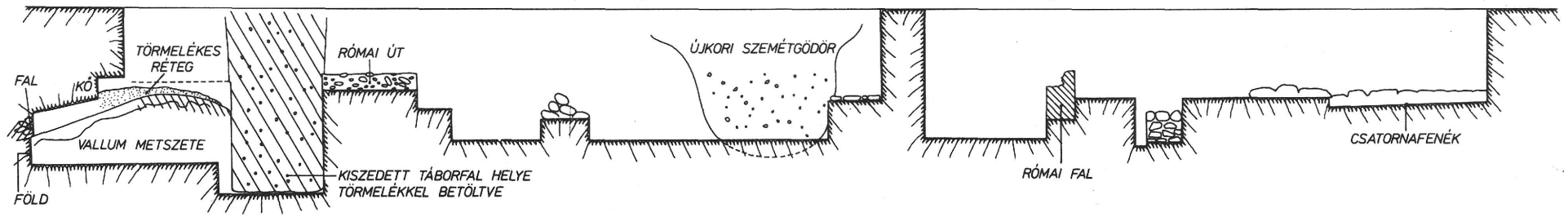
A B C D A-B METSZET B C C-D METSZET
