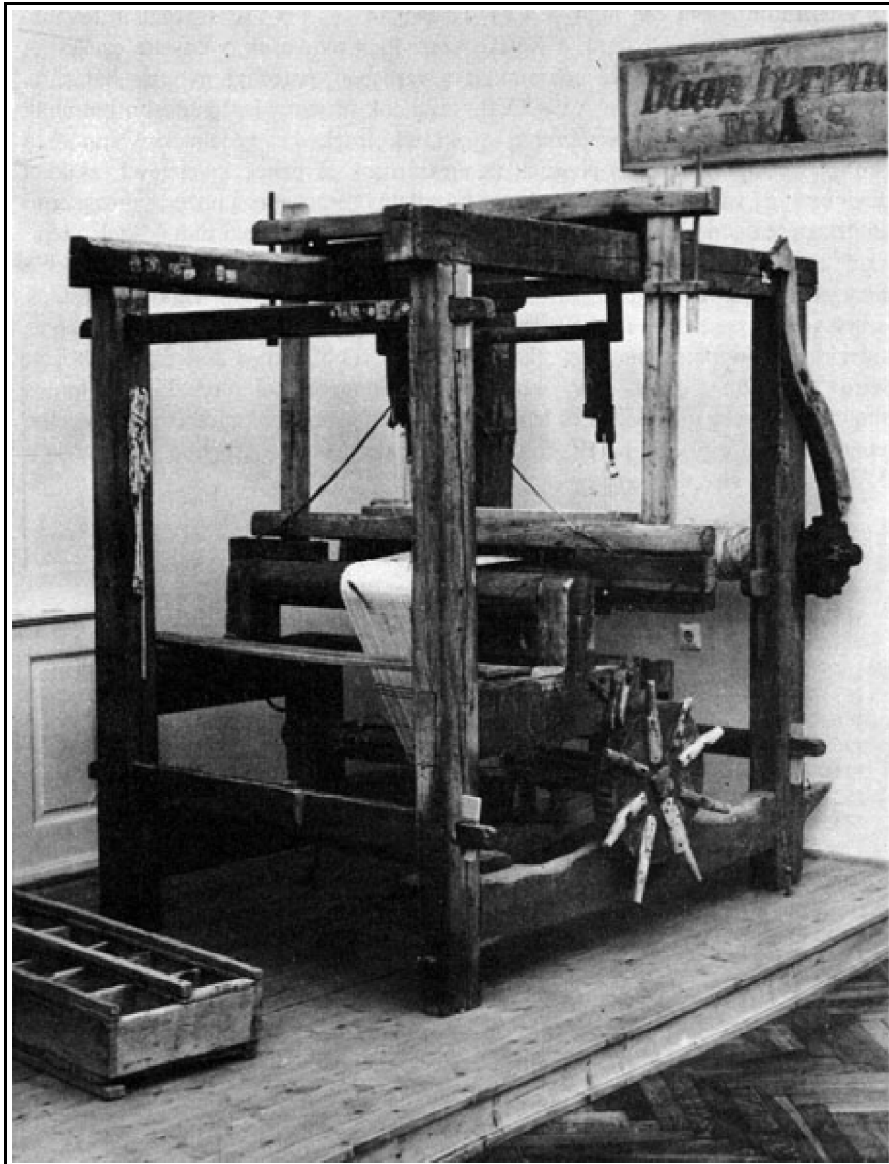
15 Gyorsvetélős szövőszék, Szakony 1891
