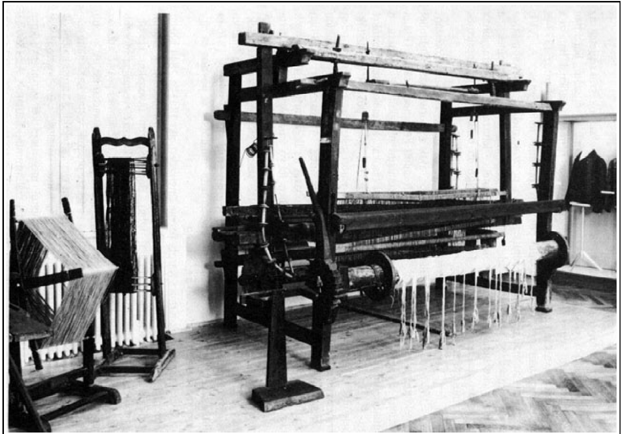
27 Kétszemélyes posztószövőszék, Krausz műhely XIX. század
