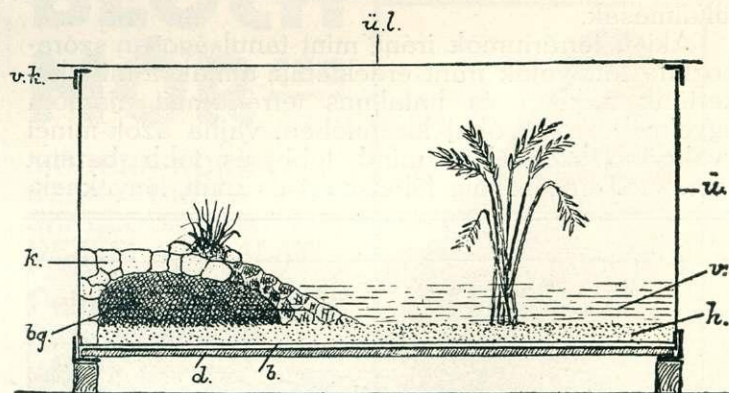
Egy aquaterrárium hosszmetezete.
