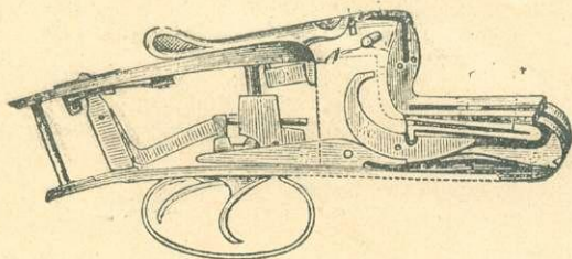
Az Anson & Deeley-féle kakas nélküli fegyver lakatszerkezete.
