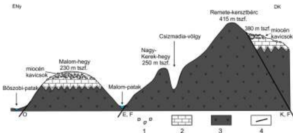
8. ábra. A kutatási terület ÉNy-DK metszete Jelmagyarázat: 1 – Kavicsok, 2 – Lajtai Mészkö Formáció, 3 – Vulkáni kőzetek, 4 – Vetők (E – ELEČKO et al. 1998, K – KÖRPÁS & CSILLAGNÉ 1999, F – FODOR 2010, O – OLÁH et al. 2014 alapján)
