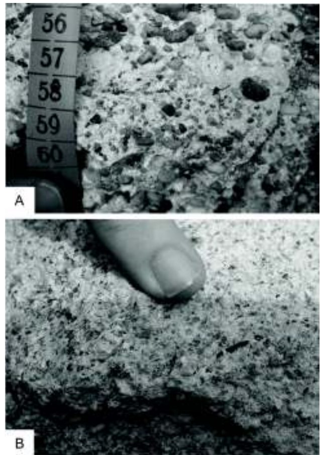
1. kép. A Lajtai Mészko kavicsos kifejlődésének makroszkópos képe. A – Osztályozatlan szemcsék (zebegényi mészko bányája), B – Jól osztályozott szemcsevázú kőzet rész (Kicsind, Köves-tető - Malá nad Hronom, Kamence).
