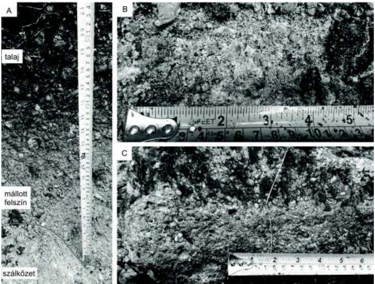
4. kép. Az RK feltárás. A – A feltárás rétegei, B – A szalkőzet nagyított képe, C – A völgyoldali helyzetű szalkőzet kibukkanása Picture 4. RK outcrop. A – layers of outcrop, B – Zoom to bedrock, C – Basset of bedrock in valley side
