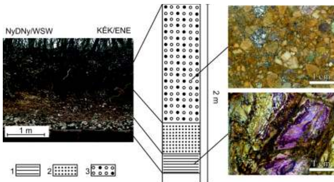
4. ábra. Az Apáthy-szikla-Kőkapu „felső-eocén báziskonglomerátum” rétegsora 1 - Foliált katakláizit; 2 - Homokkő; 3 - Oligomikt konglomerátum
