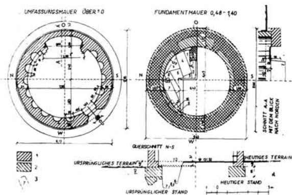
B77 - Rétunde. Grundriss und Querschnitt durch das Mauerwerk des Fundamentes
