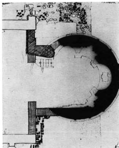
6. A karcsai körtemplom alaprajza (G. Molnár Vera nyomán)
