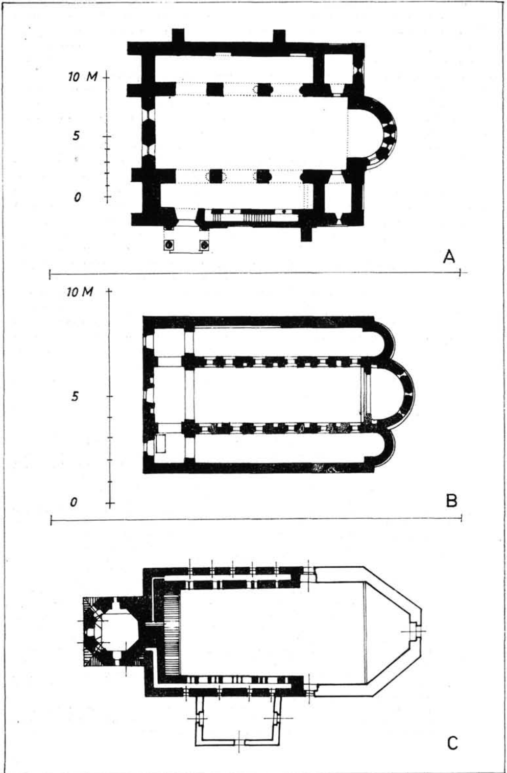
31. Templomalaprajzok: A = Boldva, B = Deáki (emeleti szint), C = Somlyóújlak
