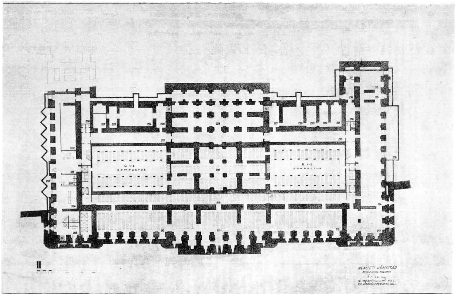
6. ábra. A II. épületszint alaprajza: raktárak, üzemek. Bal oldalon (északon) a foto- és mikrofilmlaboratórium, jobb oldalon (délen) a könyvkötészet és a sokszorosító üzem
