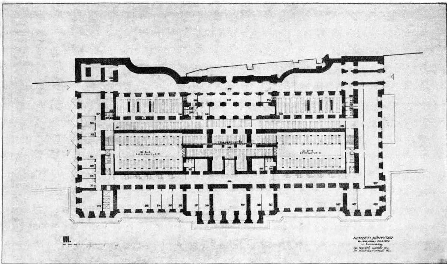
7. ábra. A III. épületszint alaprajza: bal oldalon (északon) a Csikós udvari teherkapu, mellette és az épület nyugati szárnyán a könyvforgalmi főosztály szolgálati helyiségei; a keleti szárny középső részén az angol-udvarról nyíló telefonközpont; ettől északra és délre a keleti raktárak; a déli oldalon a restauráló műhely. Középen a pontozott kettős vonal a két raktár tornyot a 4. raktári szinten összekötő könyvszállító szalagot jelzi
