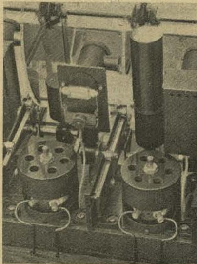
Részlet az Ericsson-gép belsejéből. Lemezek, fotocella, hanglámpa
