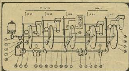
Az Ericsson-gép vázlatja
