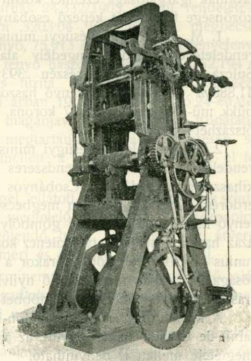
„Stell-os“ gyorskeretfűrész.
