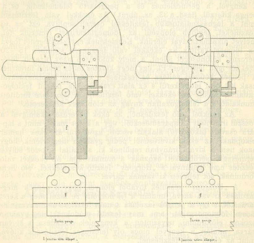
32. és 33. ábra. Horgony fűrészpenge-feszítő.
