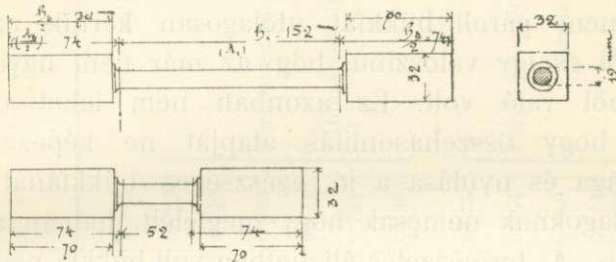
1. és 2. ábra. A próbadarabok alakja és méretei.
