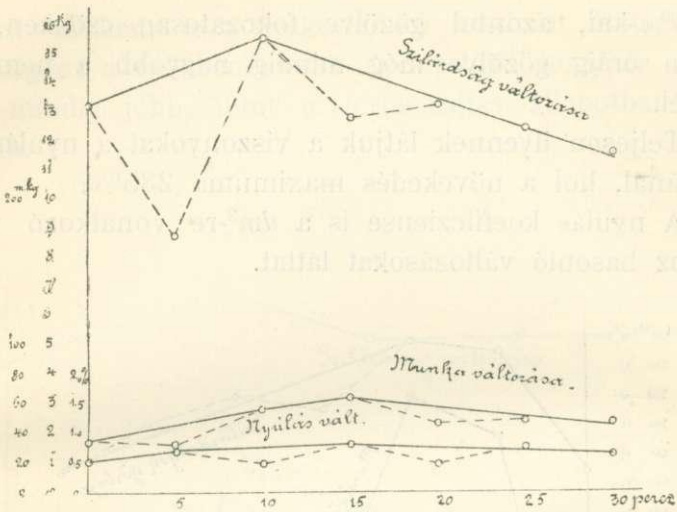
4. ábra. A 4 légk. nyomás (144° C) mellett gözzelt bükkfa egyes műszaki tulajdonságainak változását ábrázoló diagrammok.
