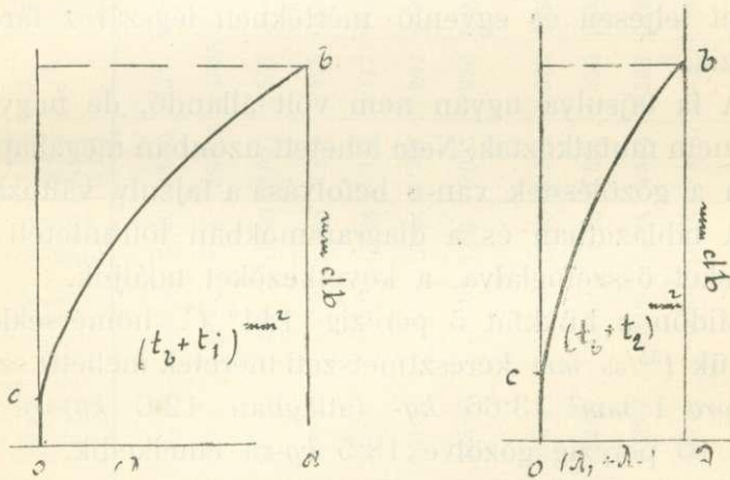
3. ábra. Az 1. és 2. ábrában föltüntetett próbadaraboknak megfelelő szakító munkadiagrammok.
