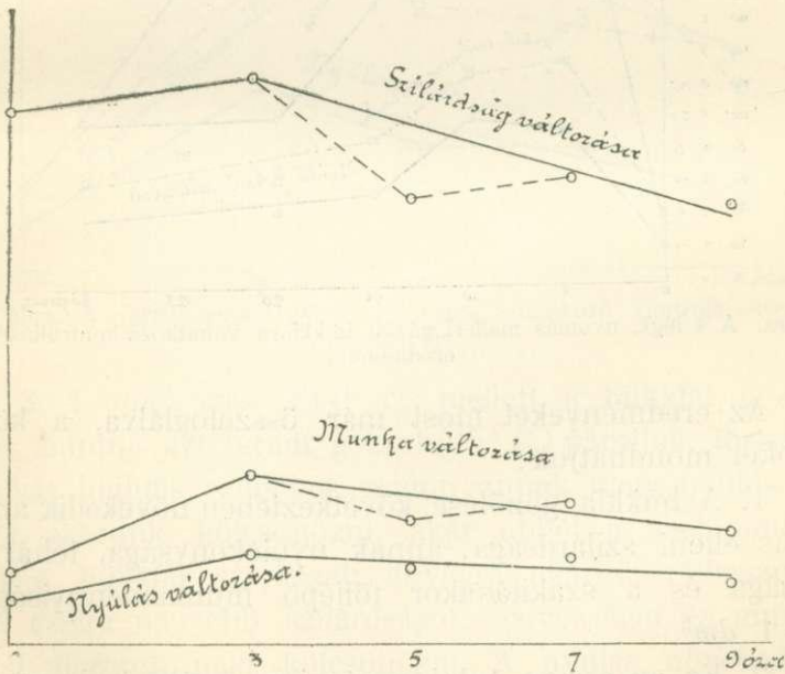
5. ábra. A fáradt (95° C) gözzel párolt bükkfa egyes műszaki tulajdonságainak változását ábrázoló diagrammok.
