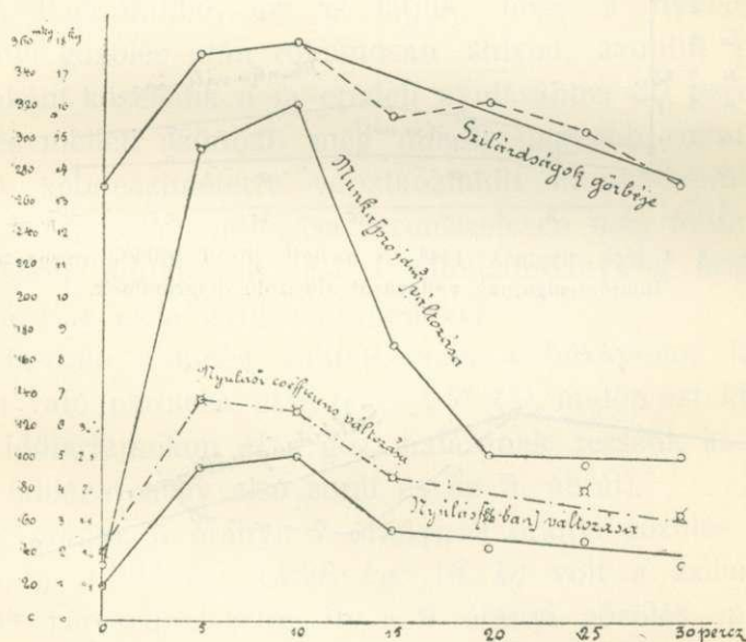
6. ábra. A 4 légk. nyomás mellett gőzölt bükkfára vonatkozó kontrollkísérletek eredményei.
