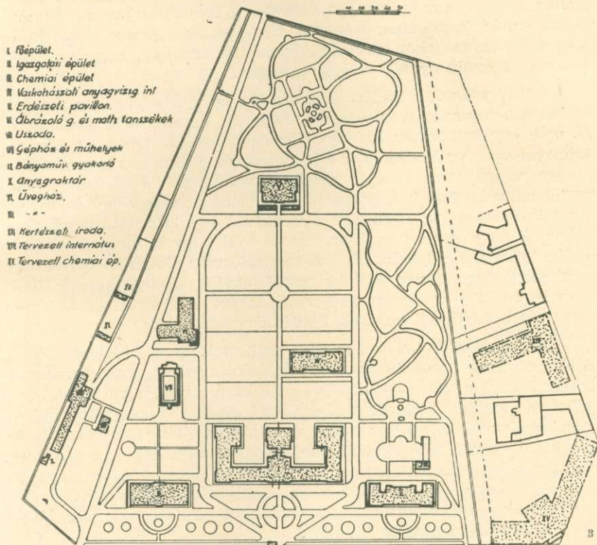
A Bányász-, Kohó- és Erdőmérnöki Kar épületének helyszínrajza Sopronban
