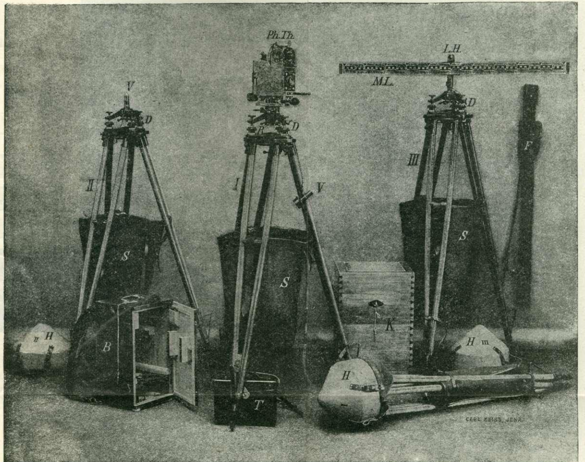
2. kép. Mezei fototheodolit és annak segítőeszközei.
