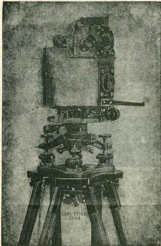
1. kép. Mezei fototheodolit.
