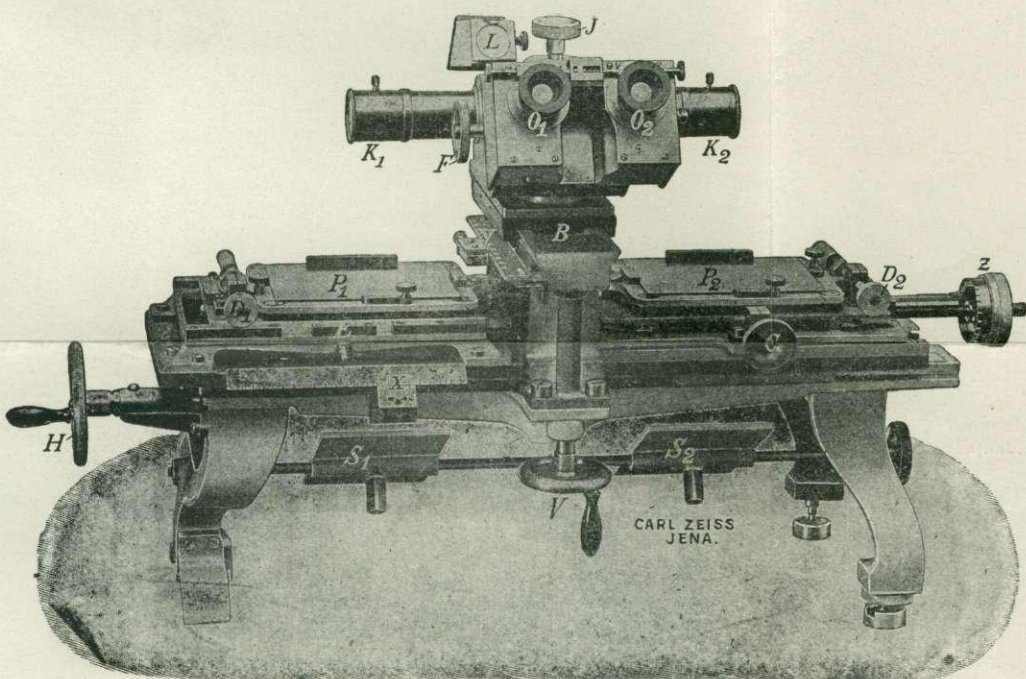
3. kép. Sztereokomparator, modell D, 9 × 12 cm-es lemezekre (1/2 természetes nagyságban).
