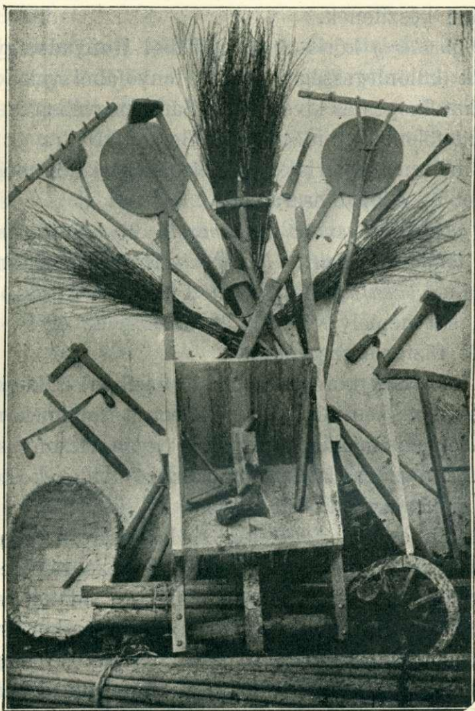
10. kép. Gazdasági eszközök és a készítésüknél használt szerszámok Ugocsa megyéből. (Pilisi Sándor tanár fölvétele alapján.)
