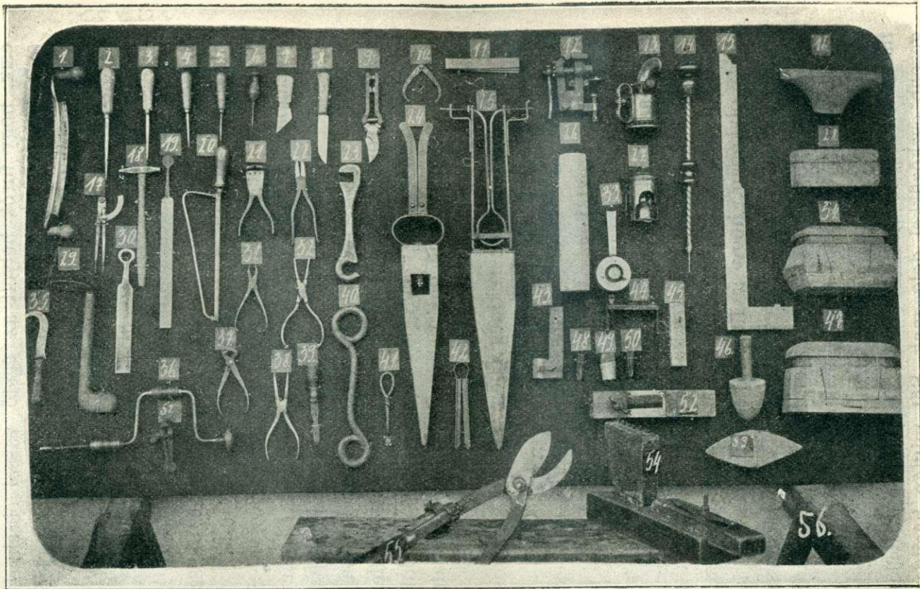
17. kép. A vesszőiparnál használt összes szerszámok. A háziiparos ezekből a készített tárgy természete szerint többet vagy kevesebbet használ. 1. szivókés, 2—6. ár, 7. bütüző, 8. faragókés, 9., 55. csiptető olló, 10. átlaló körző, 11. métermérték, 12. satu, 13. forrasztólámpa, 27. hajlítólámpa, 14. pörgettyűfuró, 15. szögellő, 16., 28., 34., 46., 47., 53. mintafák, 30 hajlítóvas, 44., 52 vesszőgyaluk, 43., 48—50. vesszőalakítók, 54. gyalupad vékonyító és keskenyítő-gyaluval, 56. munkasztal stb. (Balogh L. fölvétele.)
