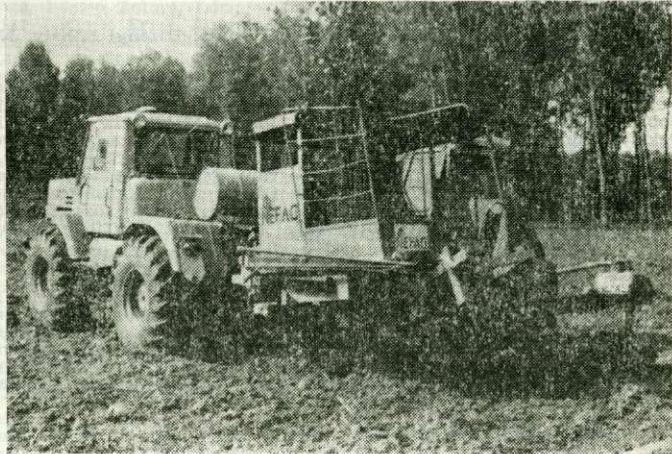
Ödörfúrásos ültetés
