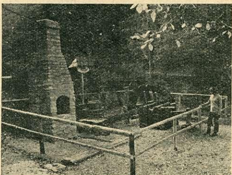
Szilvási vashámor 1790-ből
