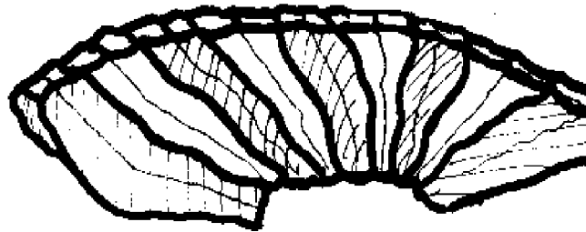
38. ábra: a kupola helyes kiterítése
