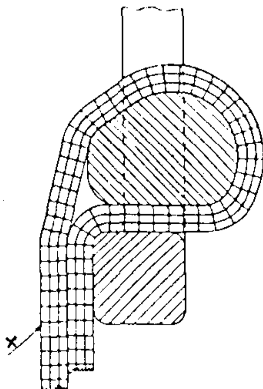
2. ábra I. típusú csúszó-rúd.
