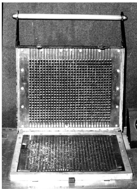
6. ábra • A számítógép programlapot leolvasó készüléke.
