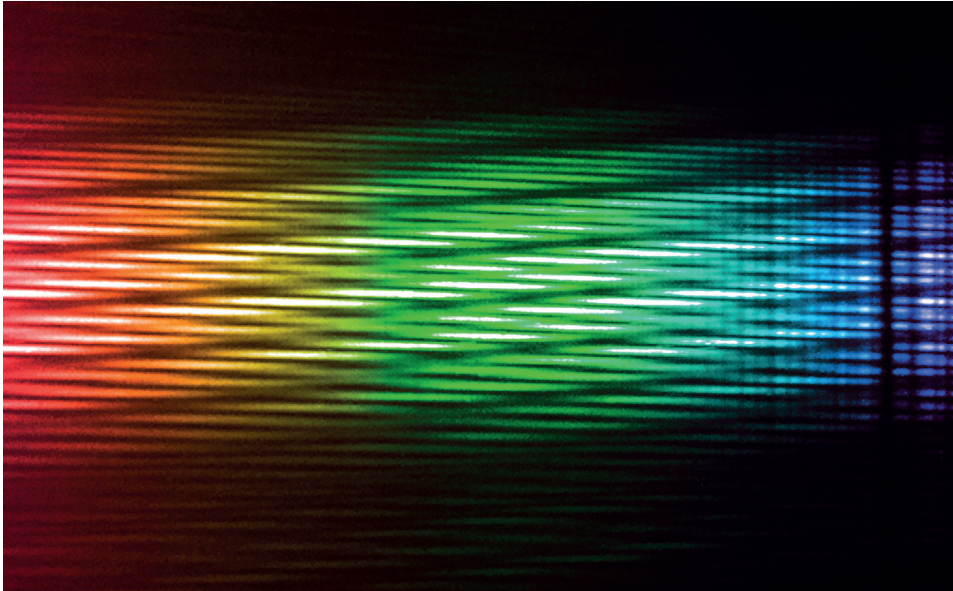
7. ábra. A Szíriusz csillagról a MATISSE-műszerrel kapott interferenciamintázat. (Forrás: ESO/MATISSE-konzorcium)
