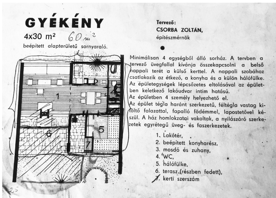
2. kép. Kézzel „áttervezett” alaprajz, Levendulás nyaralótelep, Balatonakali (a Dévényi család tulajdonában)
