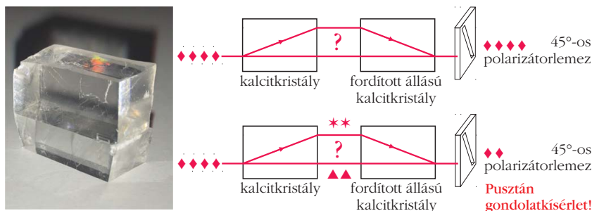
15. ábra. A bal oldali képen két, egymásra fordított állású kalcitkristályt látunk, a jobb oldali ábrán pedig a két kalcitkristállal történő egyik kísérlet sematikus rajzát. Ha feltételezhetjük (jobb alsó ábra), hogy egy foton polarizációs tulajdonsága meghatározott a két kristály között, akkor pályájukat is meg tudjuk mondani. Azonban ekkor olyan eredményt kapnánk, amelyről tudjuk, hogy téves.
