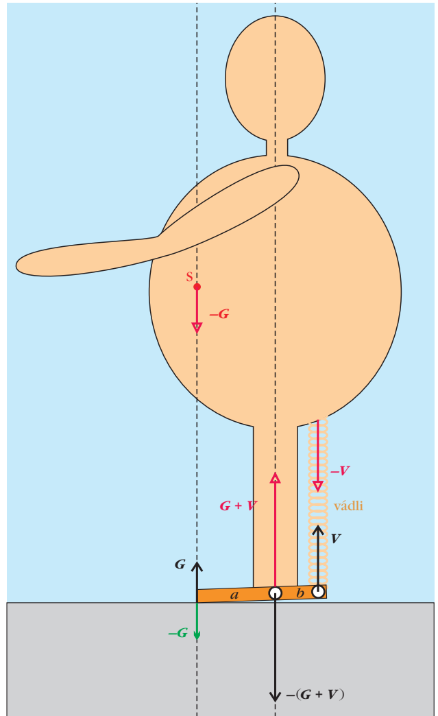
5. ábra. A sziklán stabil egyensúlyban, függőlegesen álló, sarkemelését kezdő emberre és a sziklára ható erők, amikor a test kéz-emeléssel előre mozdított „S” súlypontjának függőleges vetülete a talpcsúcson megy át, miáltal a forgatónyomaték-egyensúlyba hozott ember már nem dől hanyatt.
