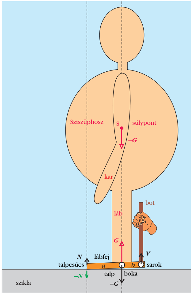
3. ábra. Egy vízszintes sziklaaljzaton stabil egyensúlyi helyzetben álló Szisüphosz-modell sarokemelését kezdő lábfejére, a test többi részére és a sziklára ható függőleges erők. N a sziklaaljzat külső nyomóereje, V a sarokot egy függőleges bottal fölfelé húzó külső erő, -G az mg/2 nagyságú fél testsúly. Az „S” súlyponton átmenő függőleges egyenes a bokát metszi. A lábfejre ható erőket v fejtű nyilak jelölik, míg a test többi részére hatókat háromszögfejtűek. A boka a láb alsó végével és a sarok a bot alsó végével forgótengellyel csatlakozik.
