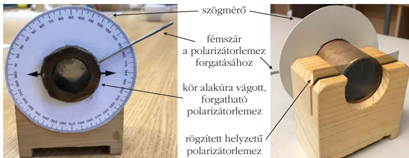
5. ábra. Az általunk használt eszköz (elől- és hátulnézetből).
