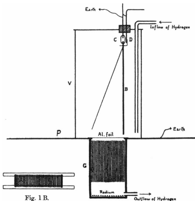
1. ábra. Rutherford első mérőberendezése az \alpha -sugarak mágneses térben történő eltérésének kimutatására [3, 179. old.].
