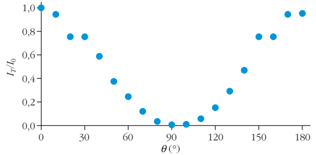
6. ábra. Az ábrán a telefonnal végzett egyik mérésünk eredménye látható. Megfigyelhető, hogy 90^\circ -nál az áthaladó fény intenzitása zérus, azaz a fény nem halad át.
