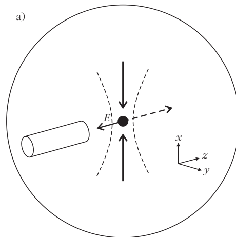
8. ábra. Elvi elrendezés nagyenergiájú ultrarövid protoncsomag (ioncsomag) hatékony előállítására (a), és a keltett deuteroncsomag energiaspektruma (b).
