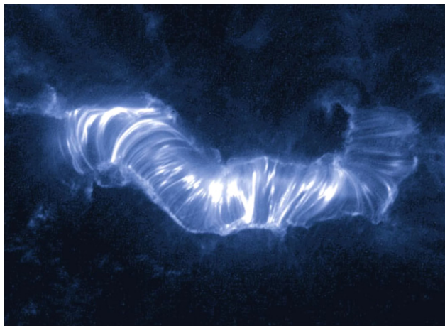
2. ábra. Mágneses hurkokból álló árkád a 2000. július 14-i fler felnyílása után a TRACE műhold felvételén (NASA).
