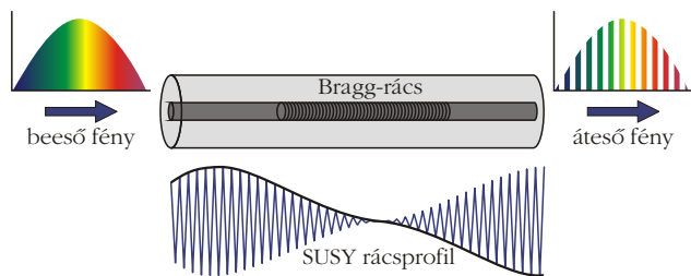
A frekvenciafésű átteresztő szűrőt megvalósító szuperszimmetrikus rácsprofil.
