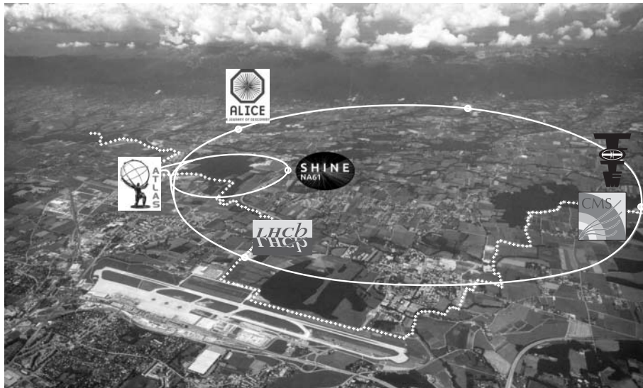
1. ábra. Légifelvétel a CERN környékéről az SPS- és LHC-gyűrűkkel és néhány kísérlettel.
