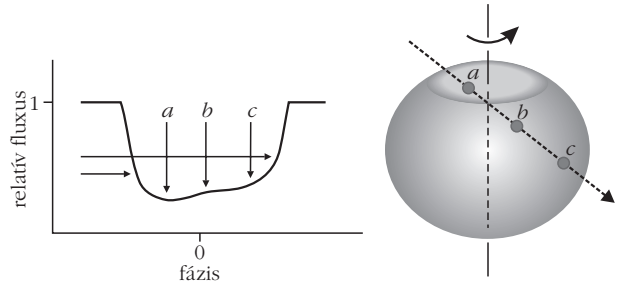
6. ábra. Torzulások egy gyorsan forgó csillag előtt áthaladó bolygó fénygörbéjén. A jobb oldali ábra szemlélteti a forgás miatt a pólusoknál kialakuló forró foltokat.
