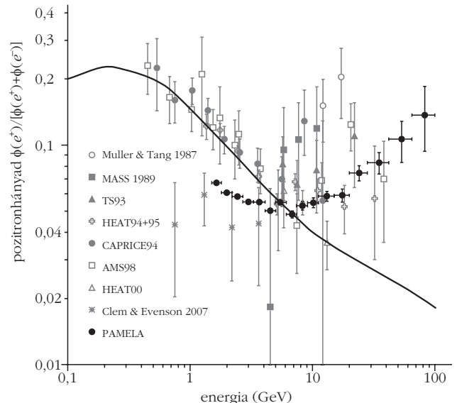
7. ábra. A PAMELA űrspektrométerrel mért energia szerinti kozmikus pozitroneloszlás egyéb korábbi mérésekkel együtt ábrázolva. A pozitronspektrum nagyenergiás szélé ellentmond a kozmikus sugárzás másodlagos keltési mechanizmusán alapuló várakozásnak (folytonos vonal).
