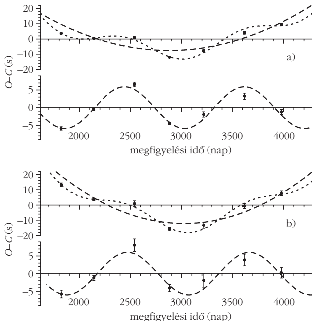
4. ábra. A V391 Peg sdB csillag O-C -görbéi a domináns és a második legnagyobb amplitúdójú módusra. A periódusnövekedés és a parabolák különbözőek. A külön bemutatott szinusz hullám mindkét esetben azonos. Egyetlen lehetséges magyarázat, hogy egy bolygó kering a csillag körül. (Silvotti et al.)
