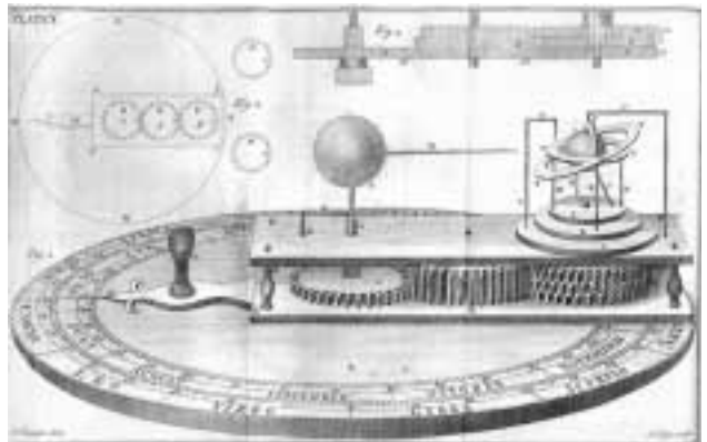
7. ábra. Cometarium-mechanizmus a 18. századból
