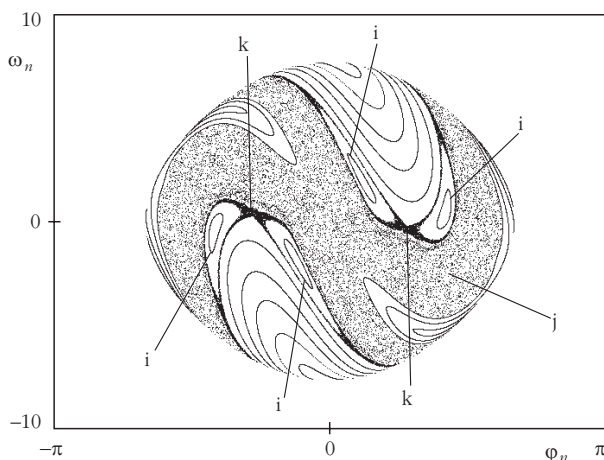
12. ábra. A 11. ábra kiegészítése Poincaré-térképpé. i -vel jelöltük a 11. ábrán látott görbéket, j -vel egy nagy, k -val egy kicsi kaotikus tartományt.
