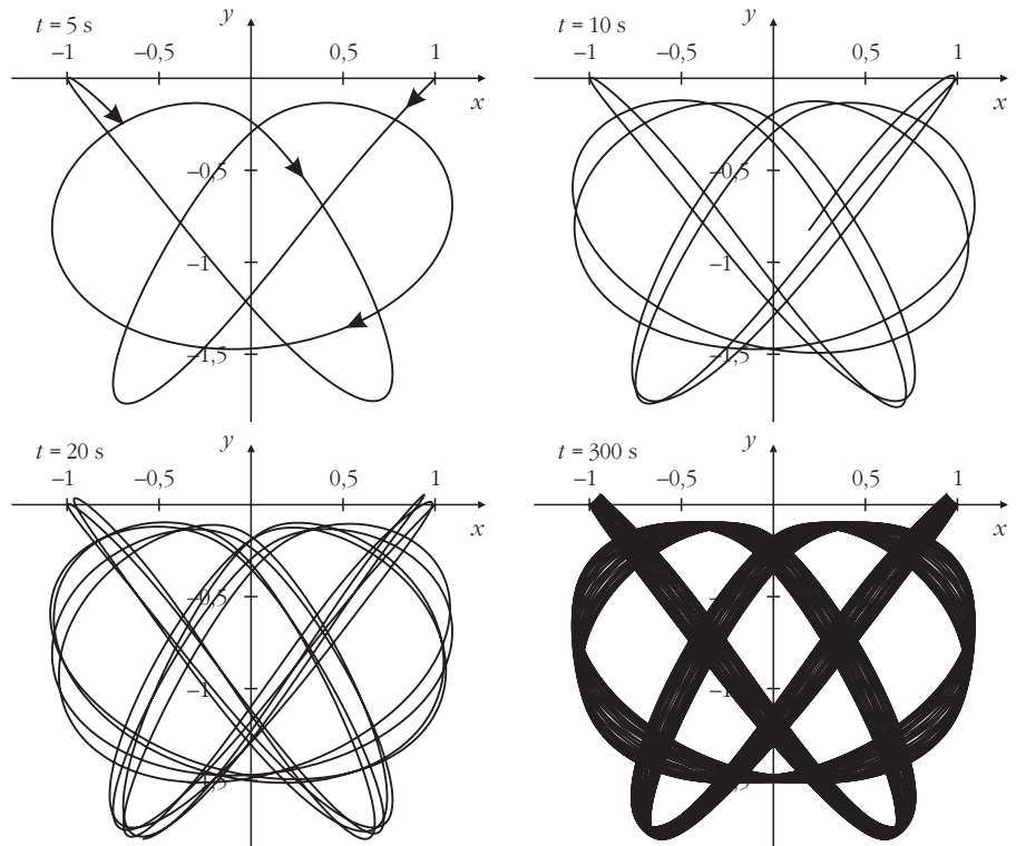
5. ábra. A 2.b és a 3.b ábra mozgásának ( m = 0,102 \text{ kg}, l_0 = 1 \text{ m} ) egyre hosszabb ideig követett pályája. Az egyes képeken leolvasható az eltelt idő. A mozgás kváziperiodikus.
