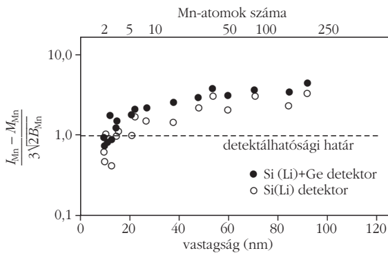
2. ábra. Az energiadiszperzív röntgenspektrométer abszolút detektálási határának függése a minta vastagságától.
