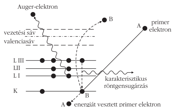
1. ábra. Analitikára alkalmas jelek elektron-besugárzáskor.
