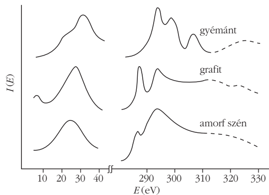
3. ábra. Szén, grafit, gyémánt EELS spektruma (R. Egerton).
