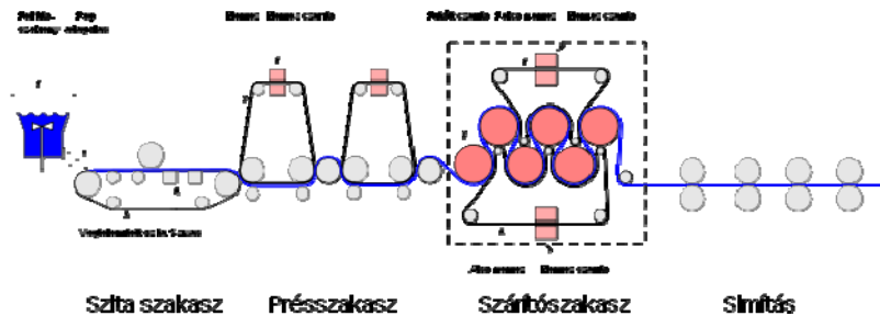
Papírgyártó gépsor vázlat
