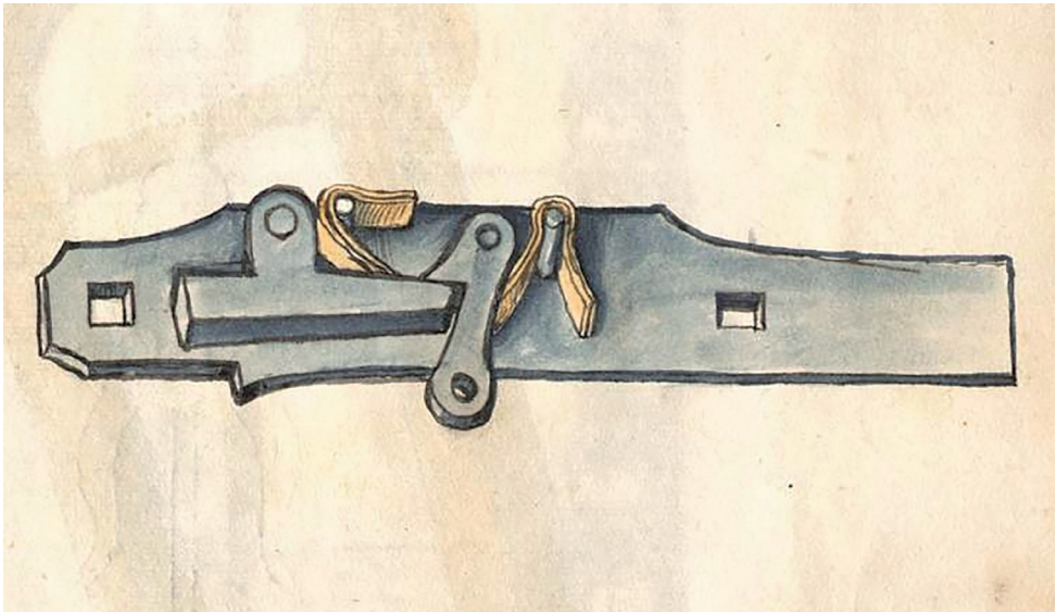
4. kép: Elsütőszerkezet Martin Merz kódexében
