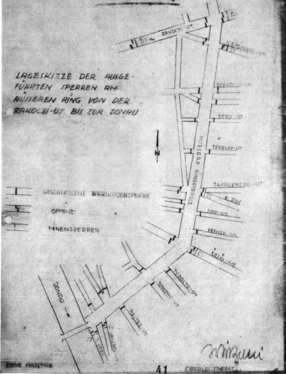
A Nagykörúton létesített műszaki záruk vázlata 2.
